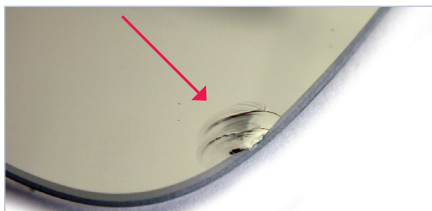
Obr. 3: Oprýskaný povlak
