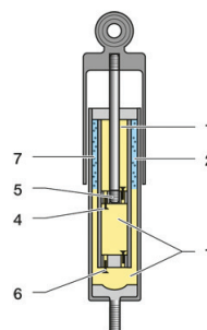
Obr. 2: Dvoupístový teleskopický tlumič nárazů
